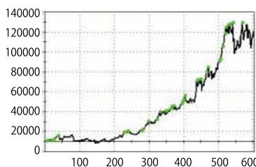
図2 オプティマル f がやや小さい
