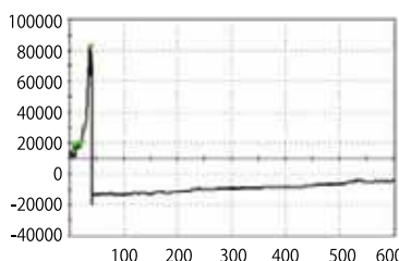
図4 オプティマル f が大きすぎる
