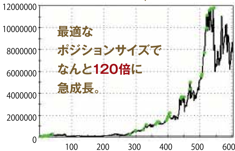
図4 オプティマル f が大きすぎる
